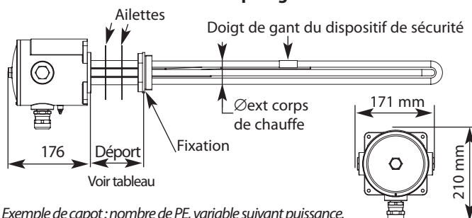
Exemple de capot : nombre de PE, variable suivant puissance.
